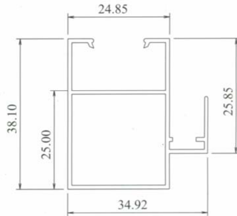
SD174 0.451 kg/m AP : 218 mm
