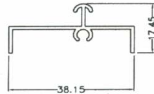
SD176 0.276 kg/m AP:167 mm
