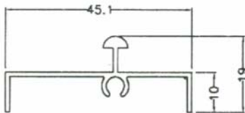
SD143 0.286 kg/m AP:182 mm
