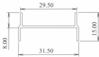
SD177 0.188 kg/m AP : 117 mm
