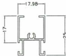
SW698 0.239 kg/m AP:185 mm
