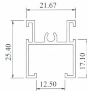
SD173 0.288 kg/m AP : 200 mm
