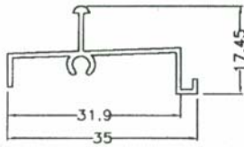
SW076 0.218 kg/m AP: 139 mm
