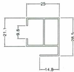
SW700 0.293 kg/m AP:180 mm
