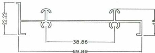
SD175 0.439 kg/m AP:309 mm
