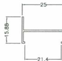
SW702 0.139 kg/m AP:115 mm
