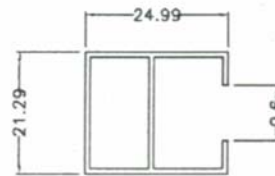
SW701 0.244 kg/m AP:1387 mm
