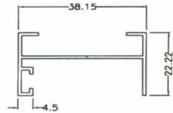
SD169 0.278 kg/m AP:203 mm
