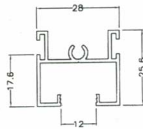
SD092 0.352 kg/m AP:242 mm
