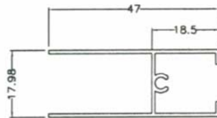
SW699 0.299 kg/m AP:249 mm
