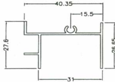
SD172 0.334 kg/m AP:220 mm
