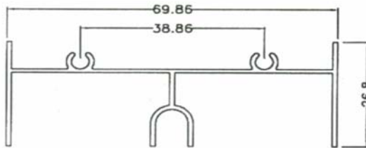
SD171 0.508 kg/m AP:342 mm
