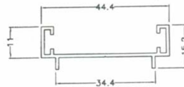
SD096 0.249 kg/m AP:176 mm
